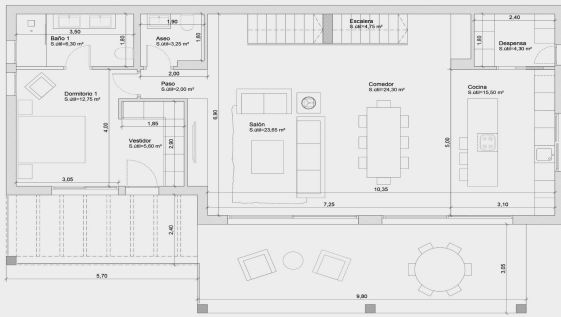
PLANTA BAJA Sup. construida vivienda 119,17 m 2 Sup. construida porche 29,90 m 2
