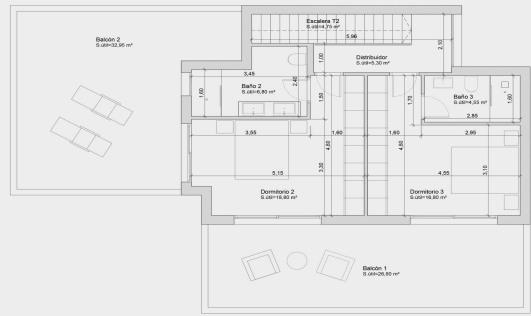
PLANTA PRIMERA Sup. construida vivienda 69,70 m 2
