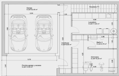
PLANTA SOTANO Sup. construida vivienda 95,43 m 2 Sup. construida porche 13,68 m 2
