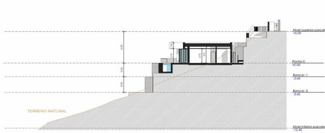
SECCIONES 01 1:200
