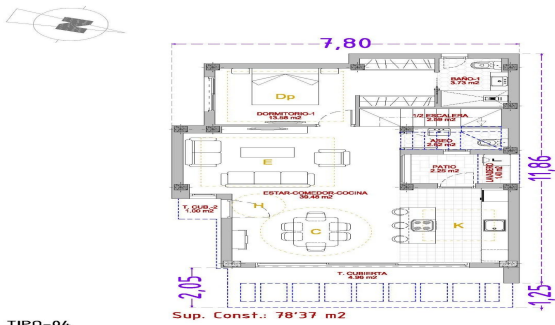
TIPO-04 VIVIENDAS Nº: 15, 16 y 17 PL/ BAJA. NOTA: El presente documento es copia de los originales del que es titular el registrante firmante del Proyecto. No sufrirá total o parcial, ni como cualquier reproducción o copia a terceros, respectivamente de la presente autorización expresa de sus autores, quedando en todo caso permitida cualquier modificación visible en el mismo.
