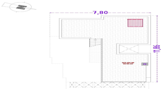
TIPO-04 VIVIENDAS Nº: 15, 16 y 17 PL/ SOLARIUM. NOTA: El presente documento es copia de los originales del que es titular el registrante firmante del Proyecto. No sufrirá total o parcial, ni como cualquier reproducción o copia a terceros, respectivamente de la presente autorización expresa de sus autores, quedando en todo caso permitida cualquier modificación visible en el mismo.
