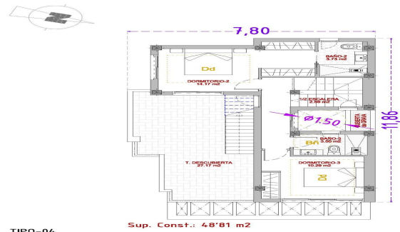
TIPO-04 VIVIENDAS Nº: 15, 16 y 17 PL/ PRIMERA. NOTA: El presente documento es copia de los originales del que es titular el registrante firmante del Proyecto. No sufrirá total o parcial, ni como cualquier reproducción o copia a terceros, respectivamente de la presente autorización expresa de sus autores, quedando en todo caso permitida cualquier modificación visible en el mismo.
