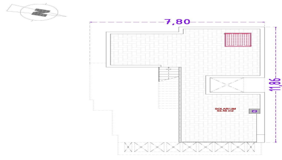
TIPO-05 VIVIENDA Nº: 18 PL/ SOLARIUM. Sup. Const.: 48'81 m2 NOTA: El presente documento es copia de su original del que es titular los arquitectos firmantes del Proyecto. No autoriza total o parcial, ni como cualquier reproducción o copia a terceros, cualquier uso de la presente documentación expresa de sus autores, quedando en todo caso prohibida cualquier modificación sustancial del mismo.
