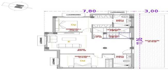
TIPO-05 VIVIENDA Nº: 18 PL/ SÓTANO. Sup. Const.: 78'06 m2 NOTA: El presente documento es copia de su original del que es titular los arquitectos firmantes del Proyecto. No autoriza total o parcial, ni como cualquier reproducción o copia a terceros, cualquier uso de la presente documentación expresa de sus autores, quedando en todo caso prohibida cualquier modificación sustancial del mismo.
