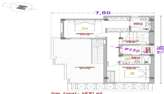
TIPO-05 VIVIENDA Nº: 18 PL/ PRIMERA. Sup. Const.: 48'81 m2 NOTA: El presente documento es copia de su original del que es titular los arquitectos firmantes del Proyecto. No autoriza total o parcial, ni como cualquier reproducción o copia a terceros, cualquier uso de la presente documentación expresa de sus autores, quedando en todo caso prohibida cualquier modificación sustancial del mismo.
