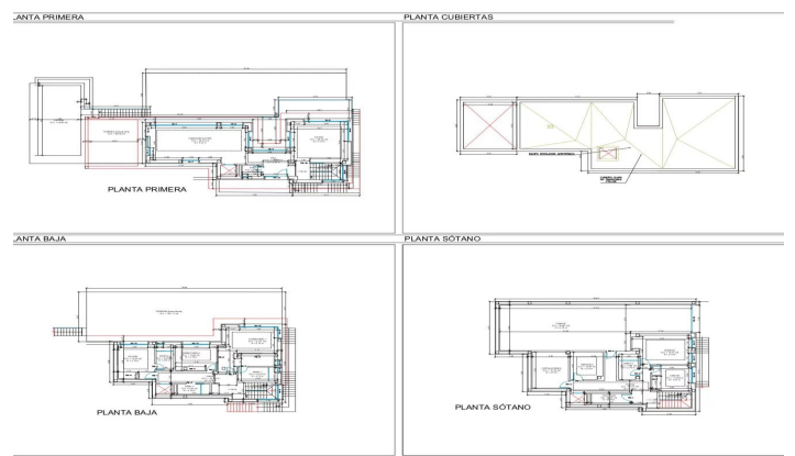
PLANTA PRIMERA
