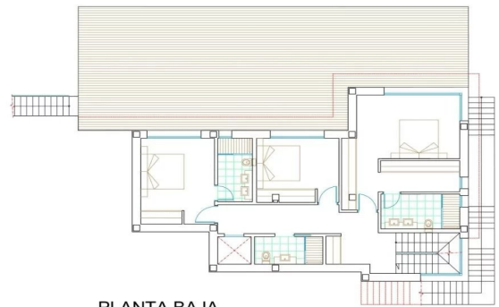
PLANTA BAJA
