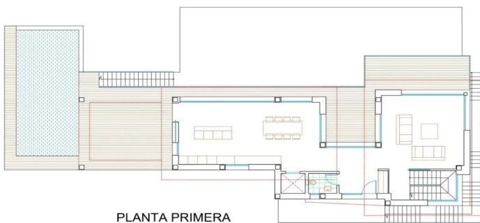
PLANTA PRIMERA
