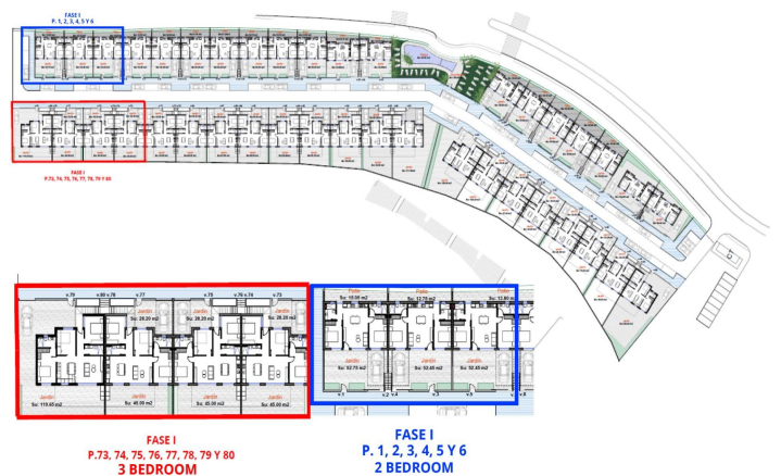
BUNGALOW TIPO Planta Baja 3 dormitorios
