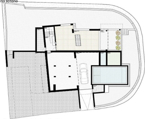
Planta sótano
