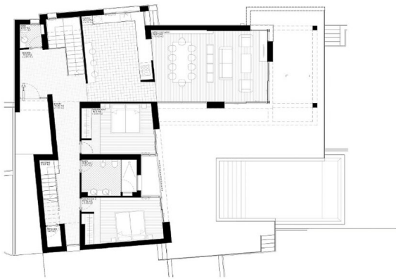
Planta sótano
