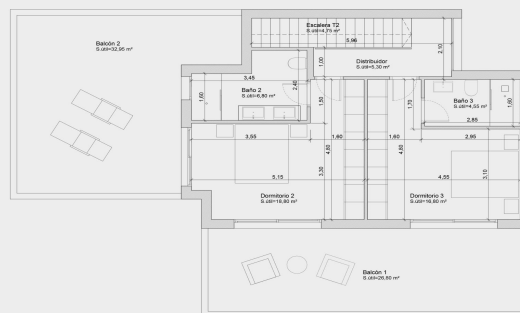
PLANTA PRIMERA Sup. construida vivienda 69,70 m²
