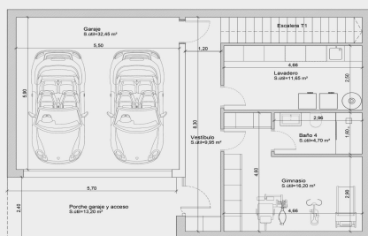
PLANTA SOTANO Sup. construida vivienda 95,43 m² Sup. construida porche 13,68 m²
