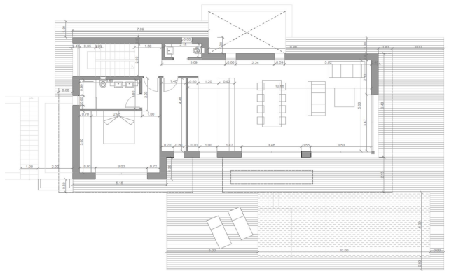
PLANTA BAJA
