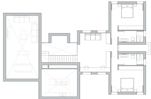
Planta Primera - Dormitorios y Estudio
