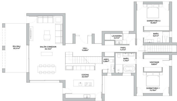
Planta Baja- Zona de día con doble altura
