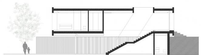
SOUTH ELEVATION ALZADO SUR
