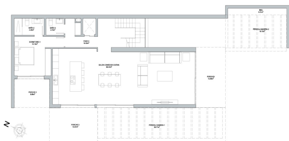
Planta Baja - Zona de día y piscina
