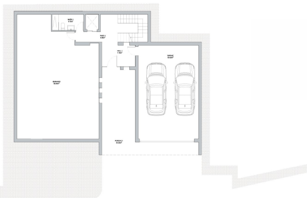
Planta Sótano - Acceso
