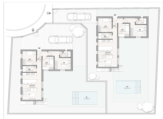
PLANTA BAJA
