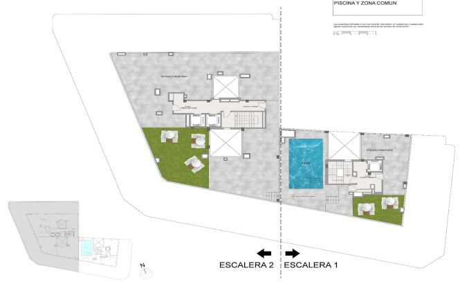
PLANTA CUBIERTA PISCINA Y ZONA COMUN
