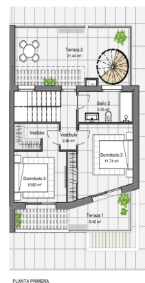
PLANTA PRIMERA
