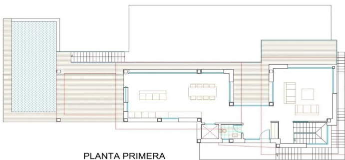
PLANTA PRIMERA
